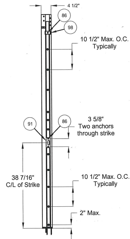
ACTIVE JAMB
