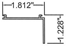
18 S/L Cap 6063-T5
