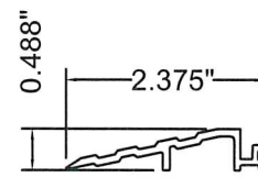
5 Leadup 6063-T5
