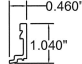
23 1" Snap 6063-T6
