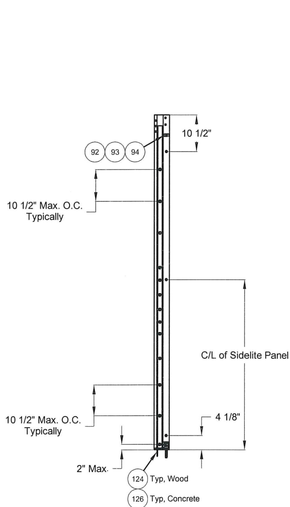
SIDELITE JAMB
