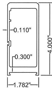
16 V2M 6063-T5
