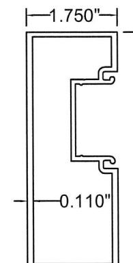
26 Jamb 6063-T6
