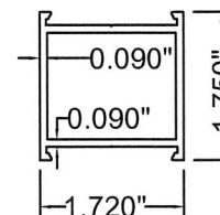
8 H2 6063-T5
