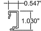
24 9/16" Snap 6063-T5
