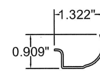
2 Sweep Clip 6063-T5
