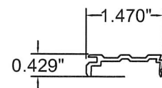
6 Filler 6063-T5
