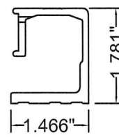
4 G-Channel 6063-T5
